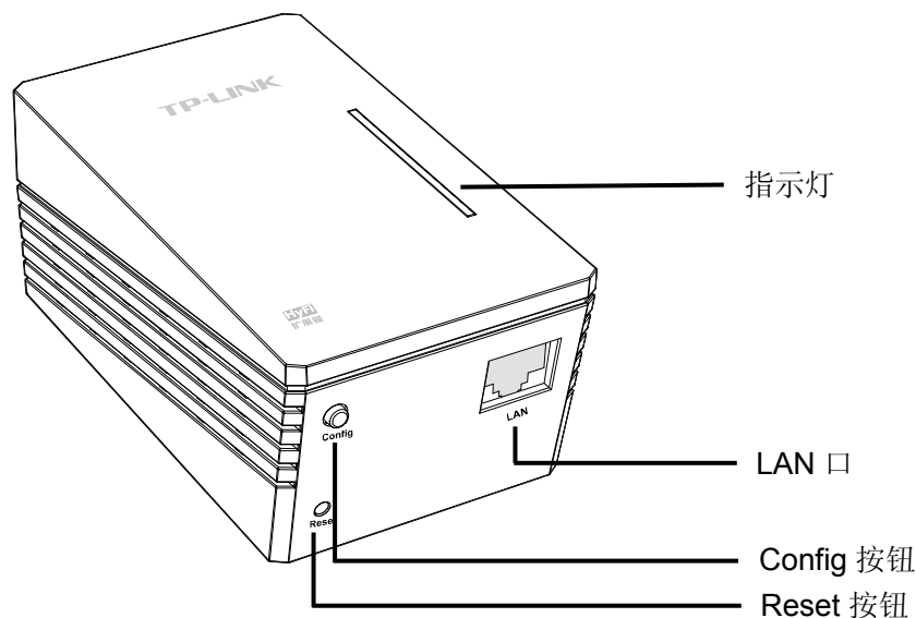
图 3-2 TL-H28E 示意图
