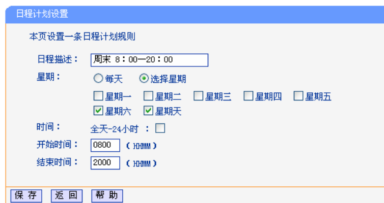
图 5-46 日程计划设置示例
