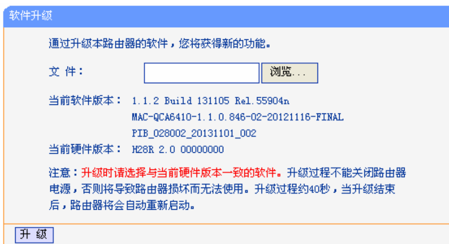
图 5-64 软件升级
