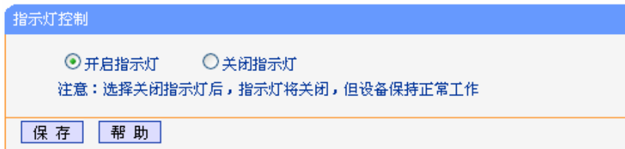
图 5-58 指示灯控制
