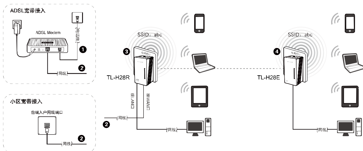
图 4-1 硬件安装示意图
