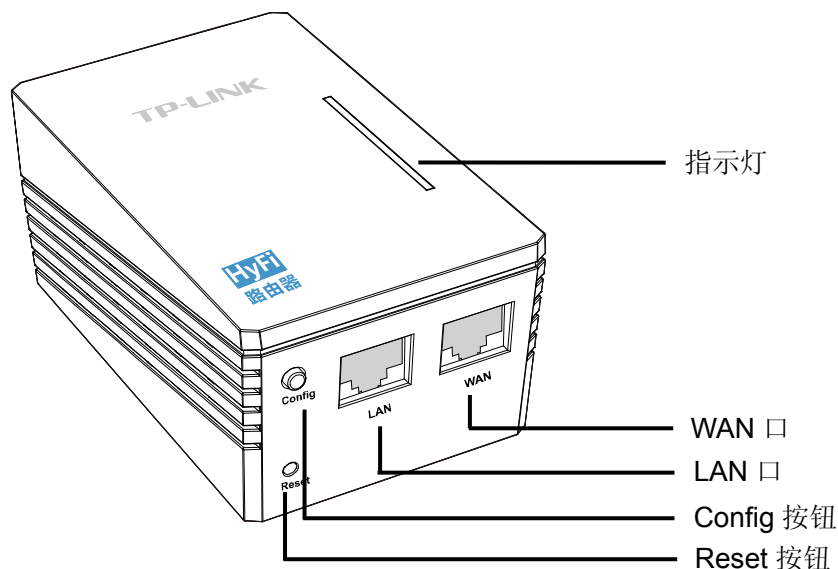
图 3-1 TL-H28R 示意图
