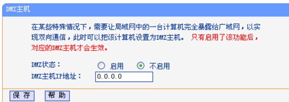
图 5-27 DMZ 主机
