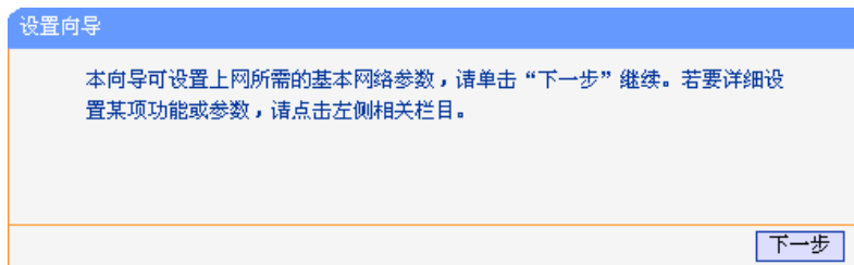
图 4-3 设置向导
