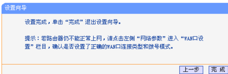
图 4-8 设置完成
