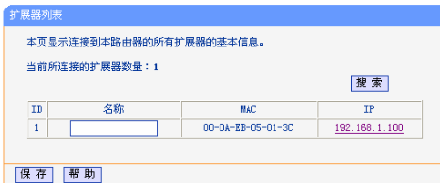
图 5-20 扩展器列表
